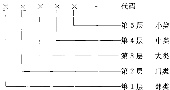
图1 代码结构
